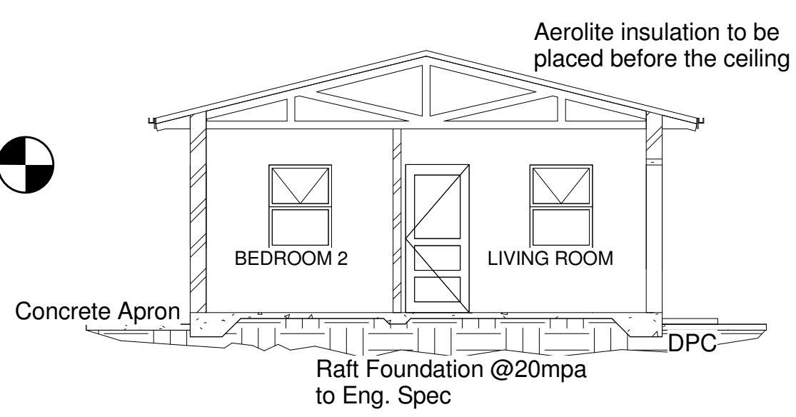
6 SECTION I 1 : 100
